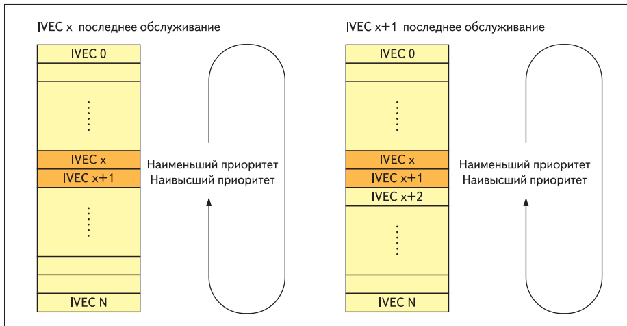
Рис. 2. Процедура «карусельной диспетчеризации» Round Robin
